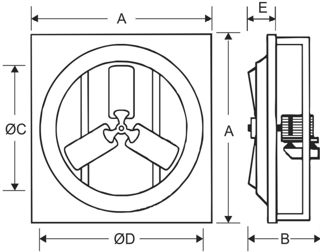
DIMENSIONES GENERALES (Dimensions)
